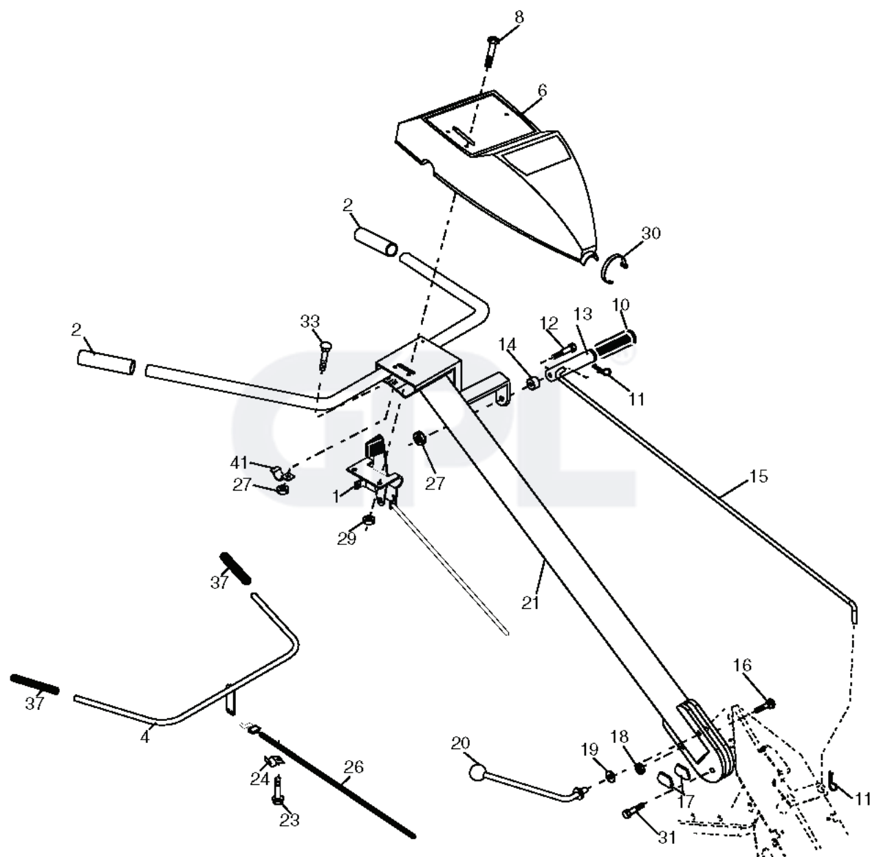
Handle_assy_99_19
