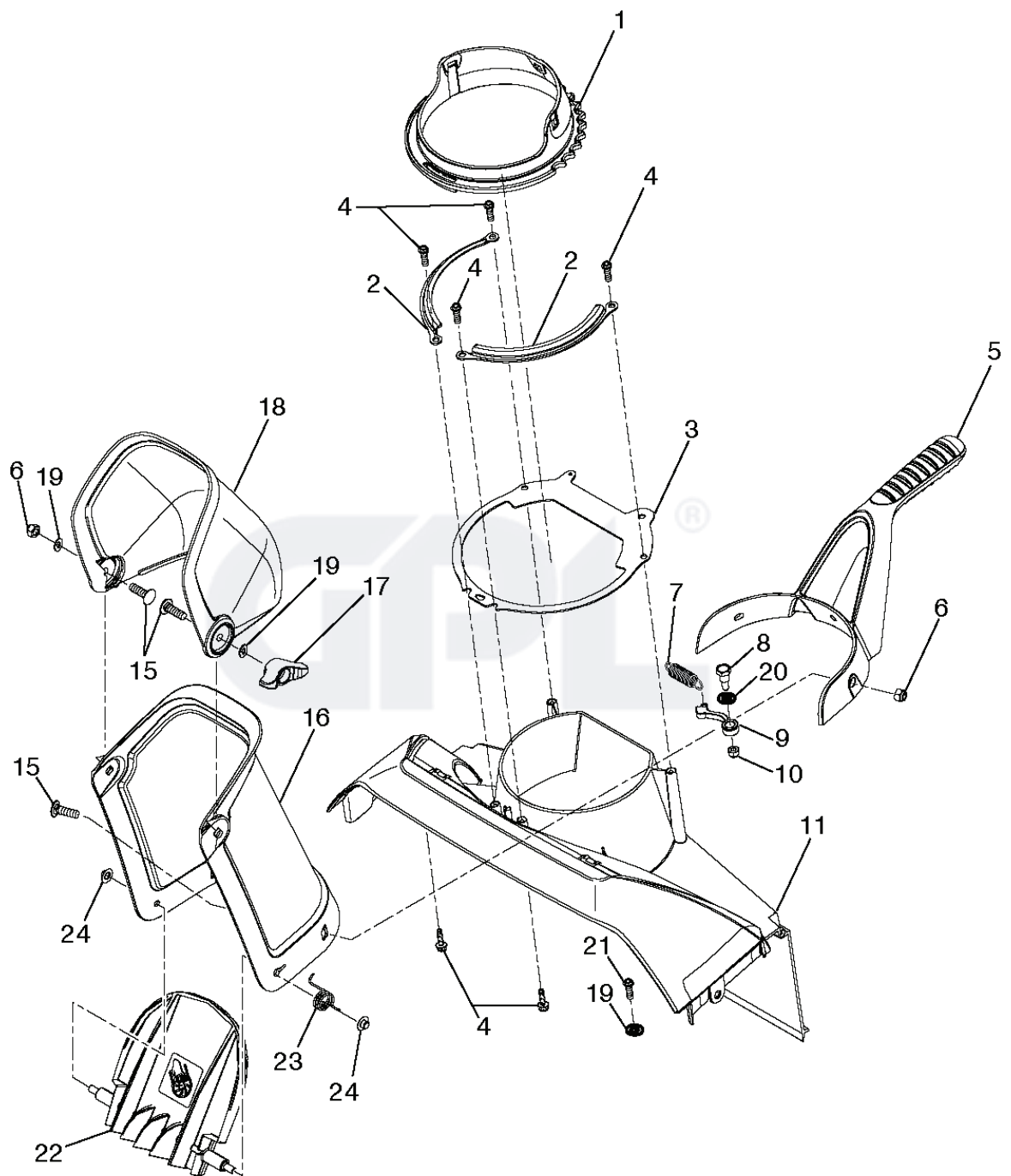
SSST-Chute asm_6
